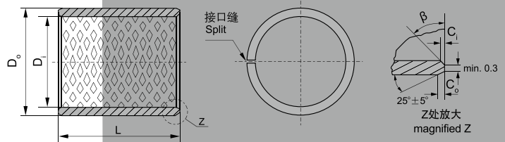
内外倒角 ID and OD chamfers
